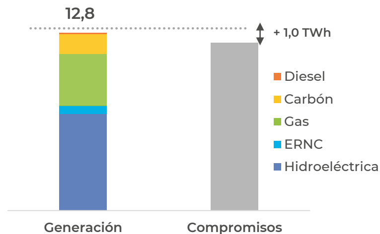
Balace de Generación vs. Compromisos Proyectados para 2023 (TWh) (2)
