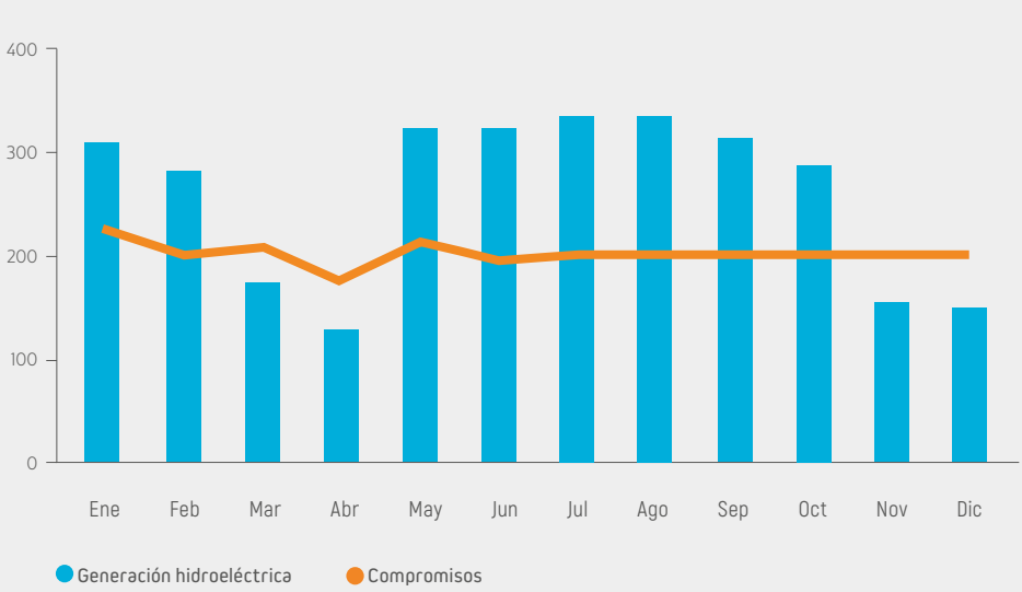
Generación Versus Compromisos 2020 (GWh)
