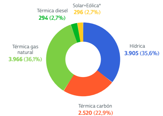
GENERACIÓN DE ENERGÍA POR TECNOLOGÍA (GWh)
